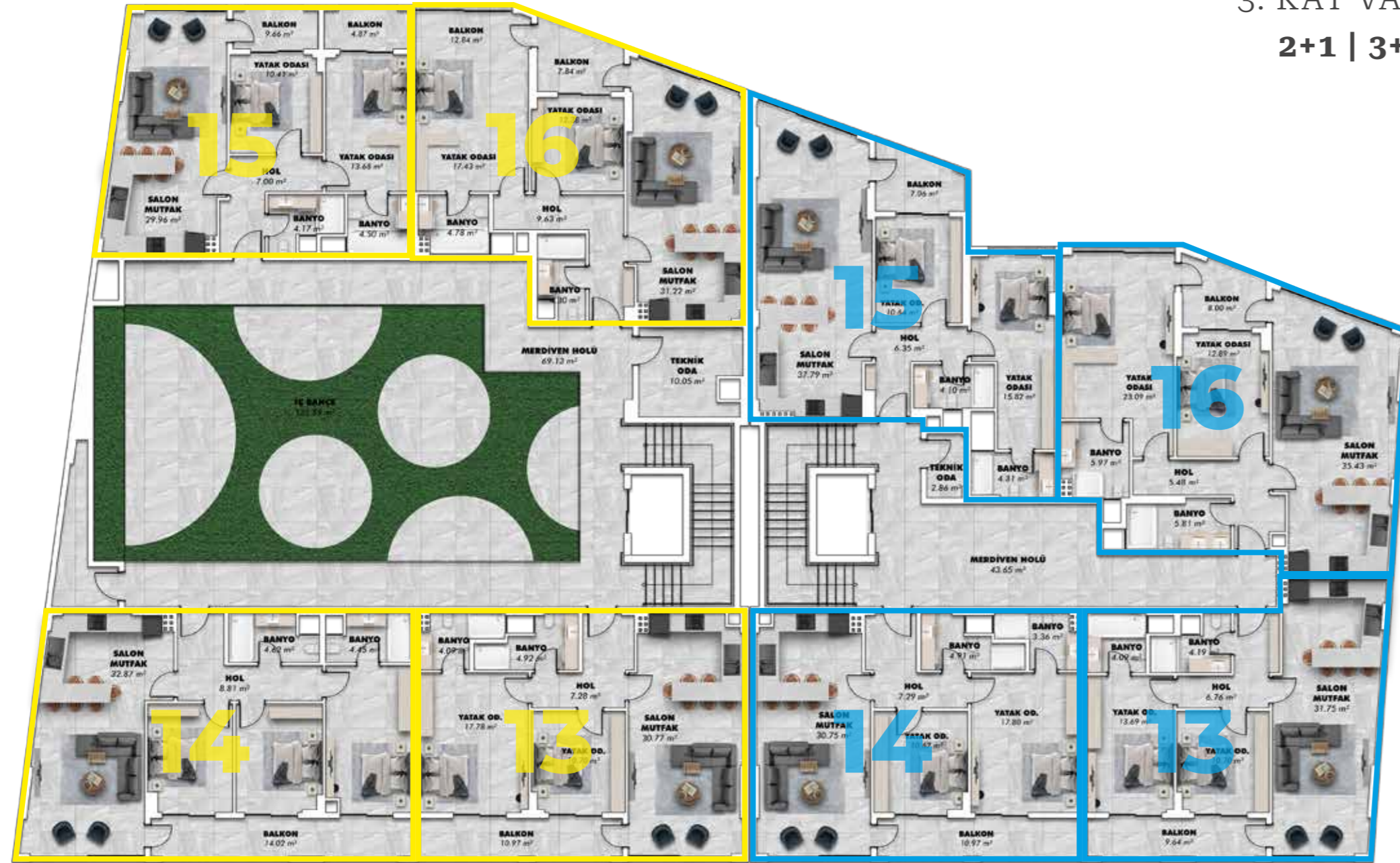
A BLOK
